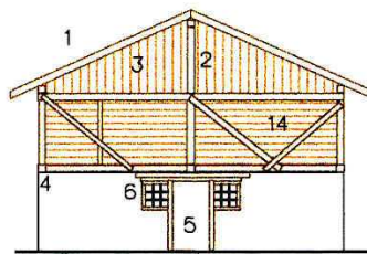
Fronte principale
